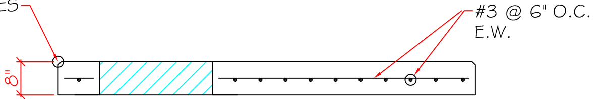
ELEVATION
